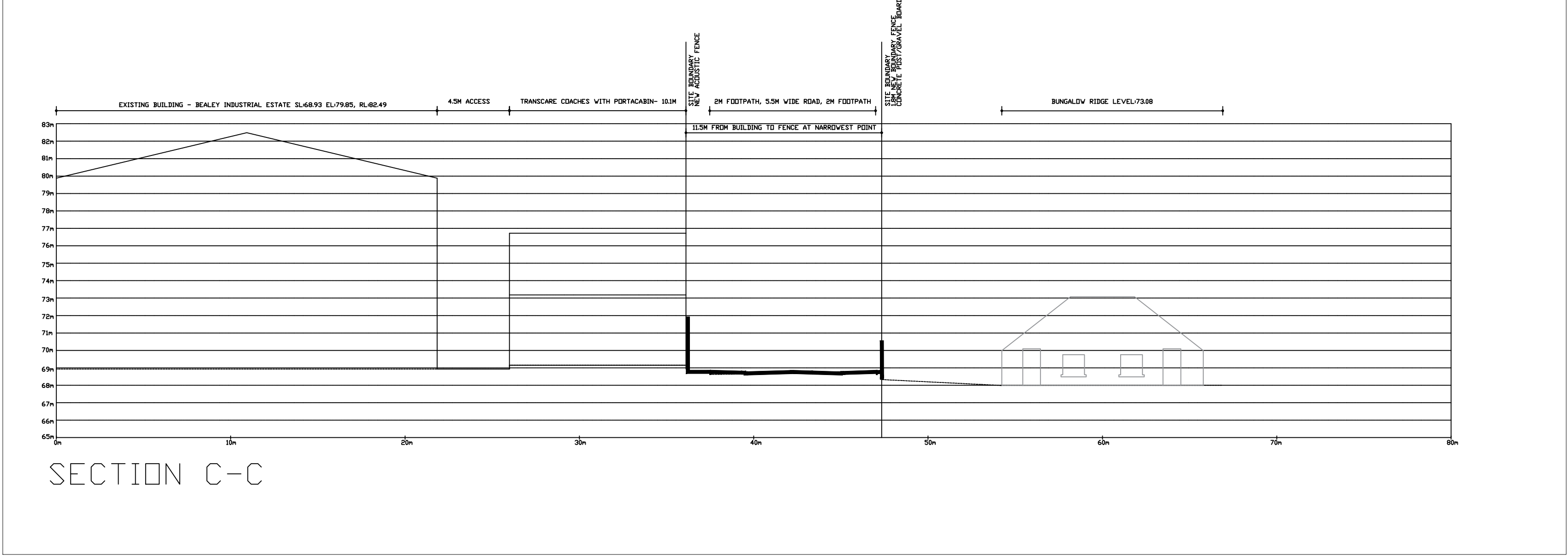
SECTION C-C SCALE-1:200
