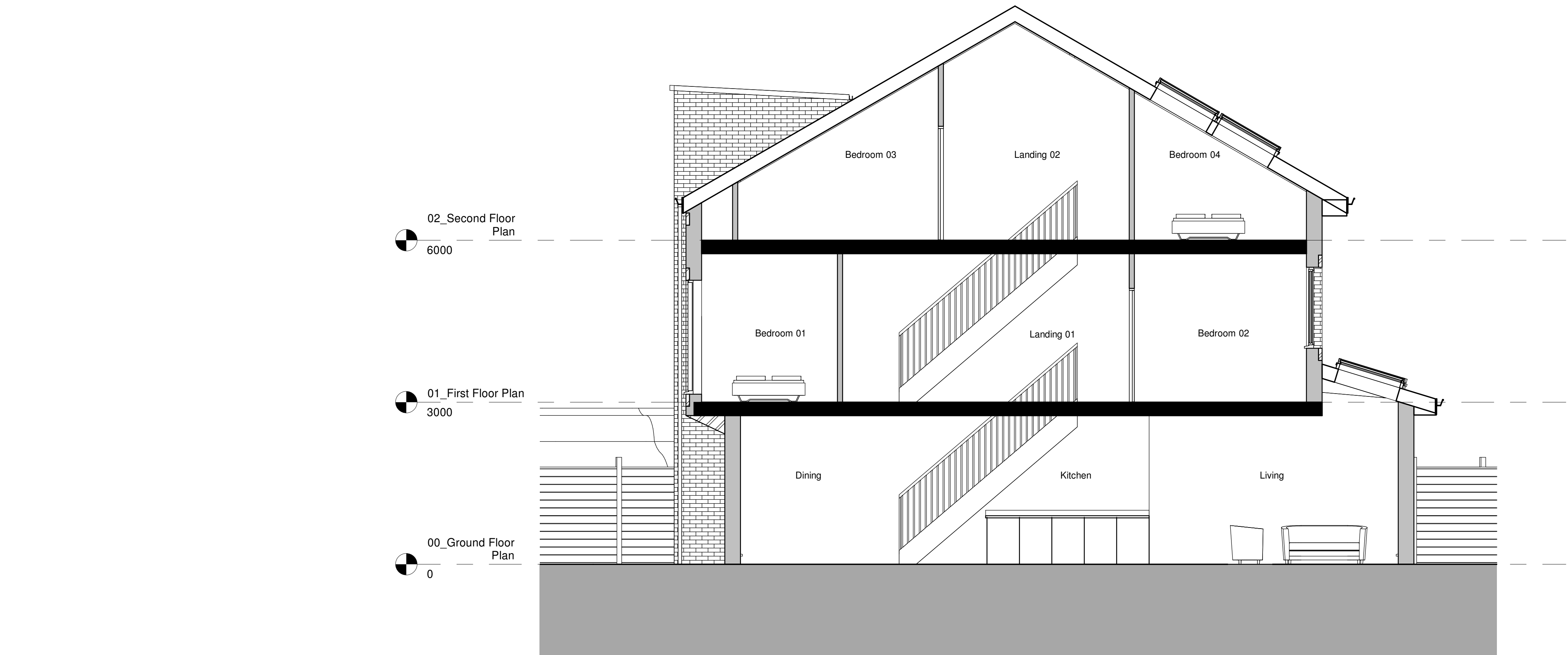
Section 1 1 : 50
