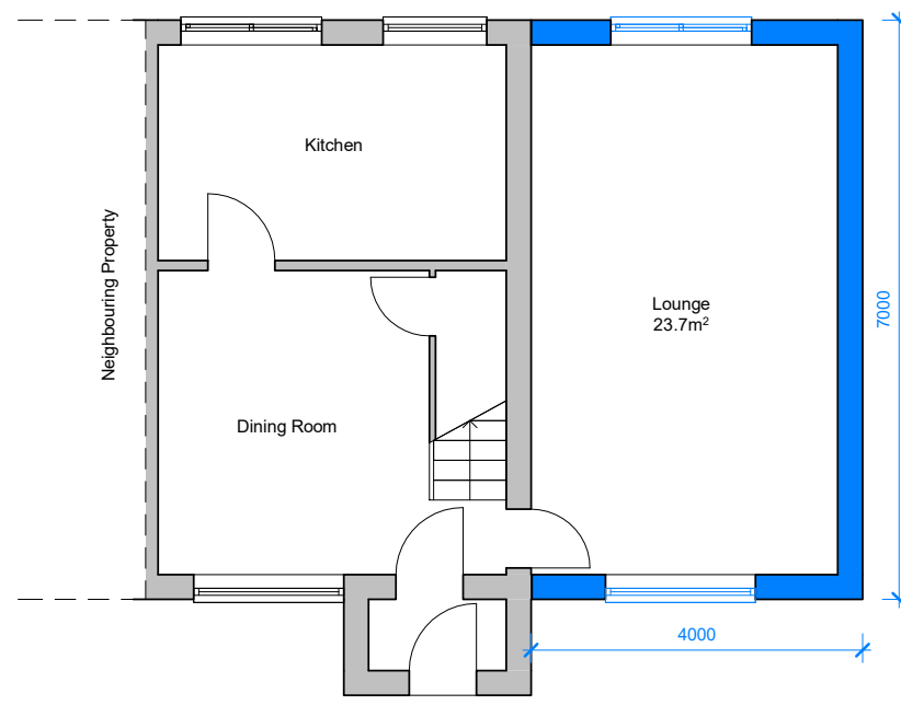
1 Level 0 1 : 100
