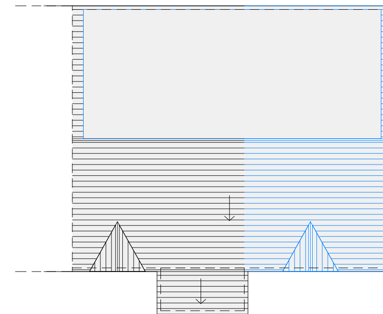
3 Roof Plan 1 : 100
