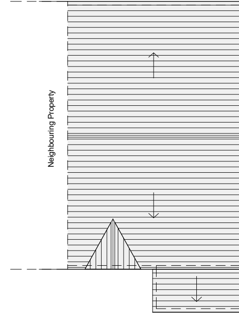
3 Roof Plan 1 : 100
