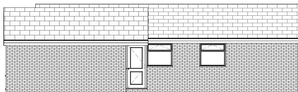
4 Garage Elevation 1 : 100
