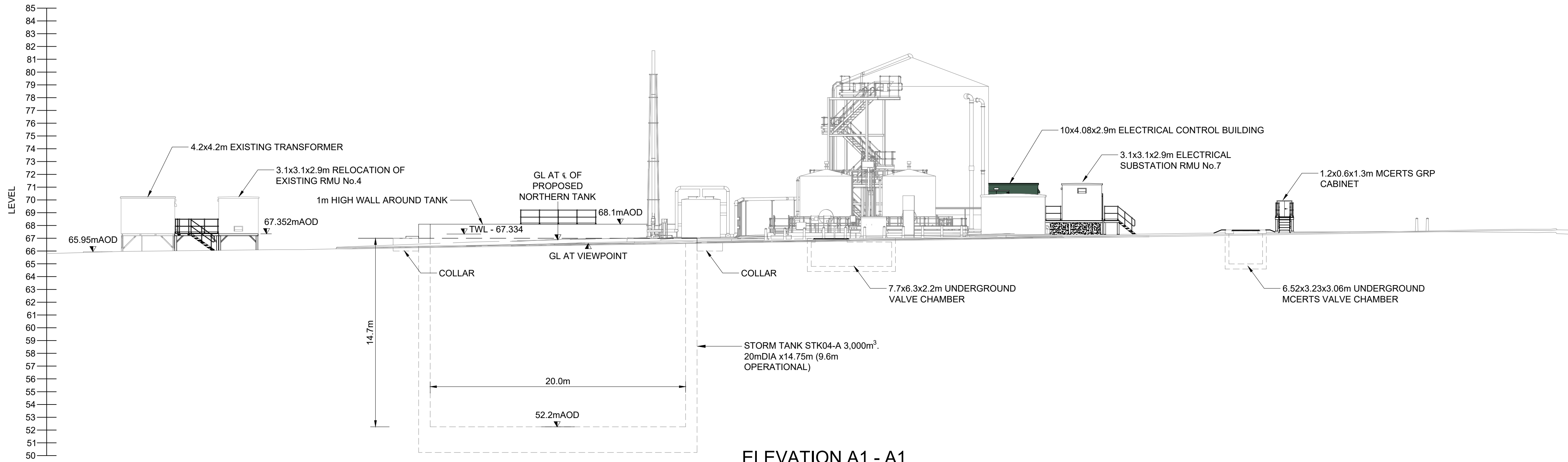
ELEVATION A1 - A1
