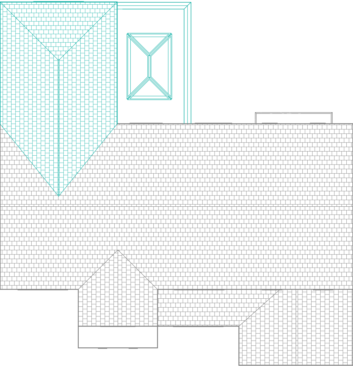
PP Roof Plan 1 : 100
