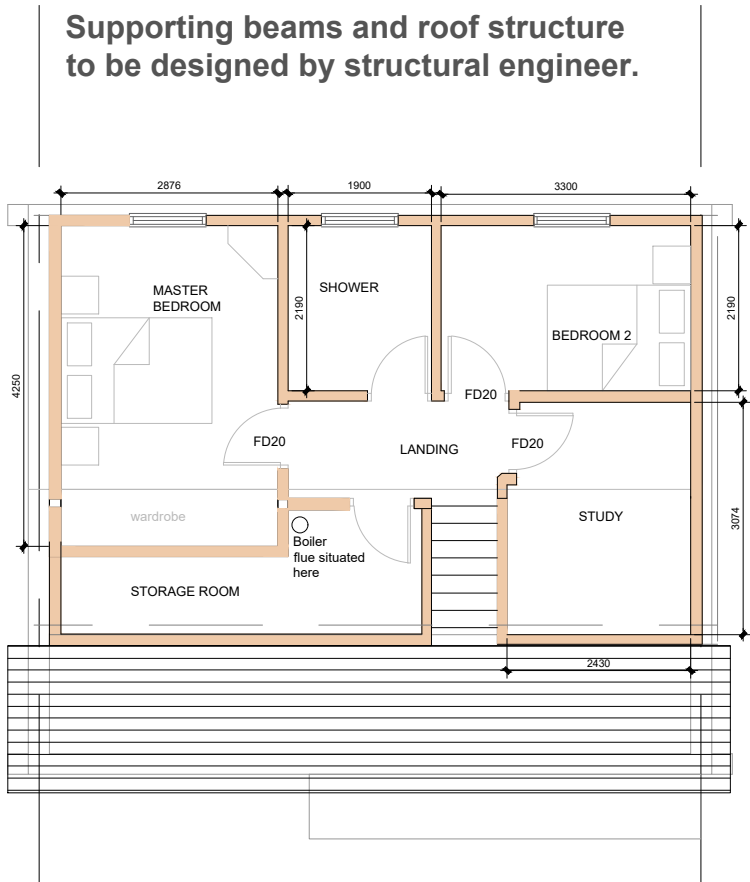
Loft Plan
