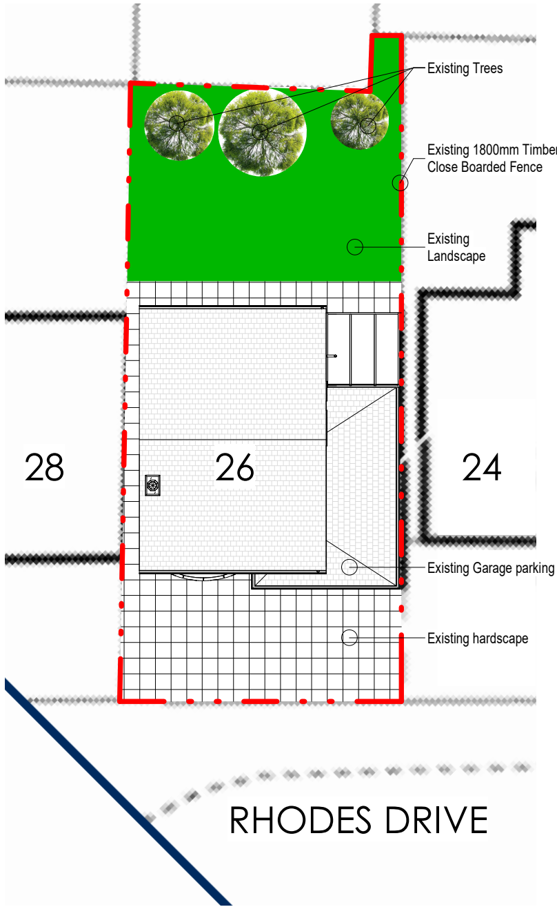
Existing Site Layout Plan 1 : 200
