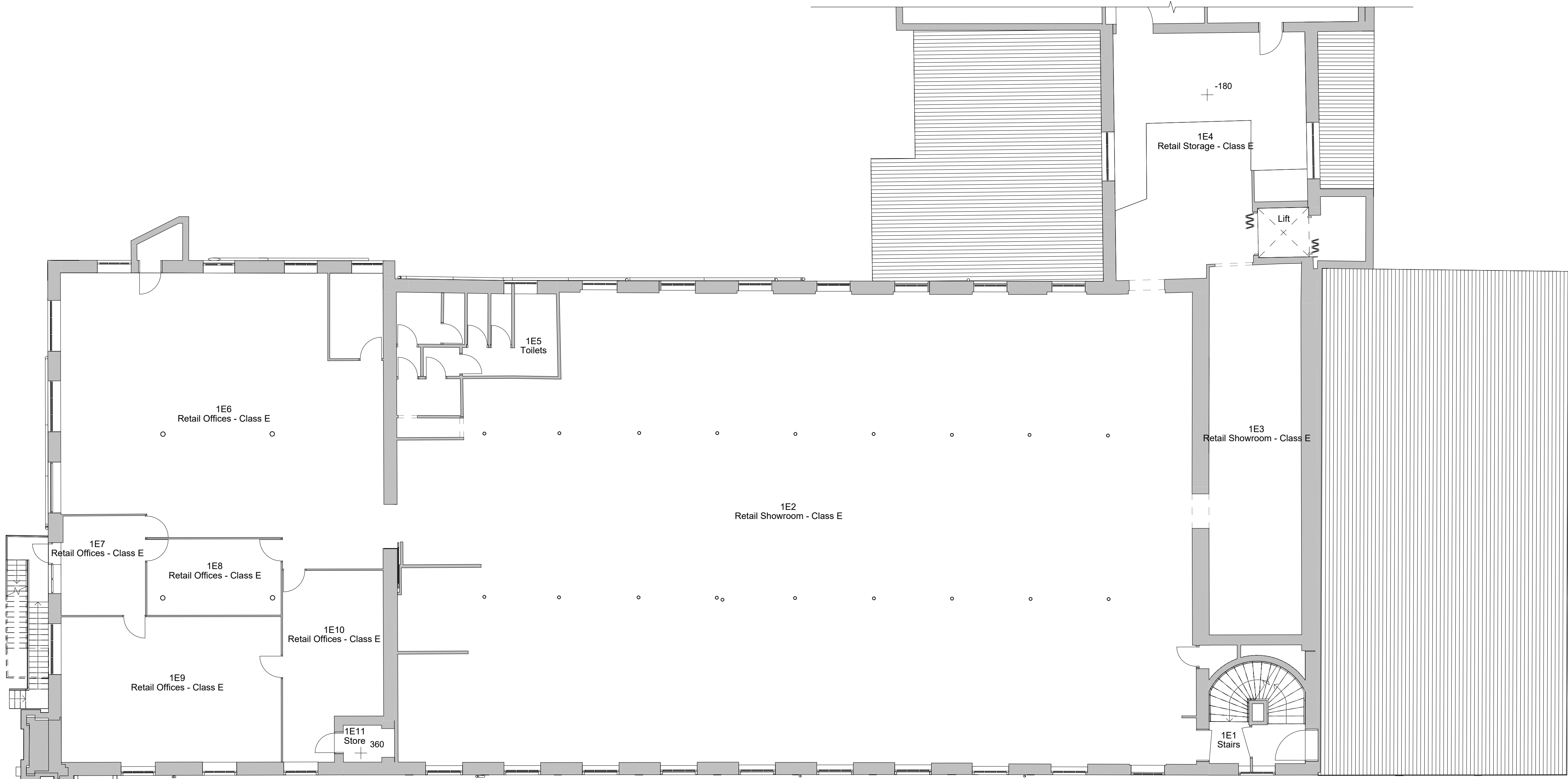
1 Level 1 - Existing 1 : 100
