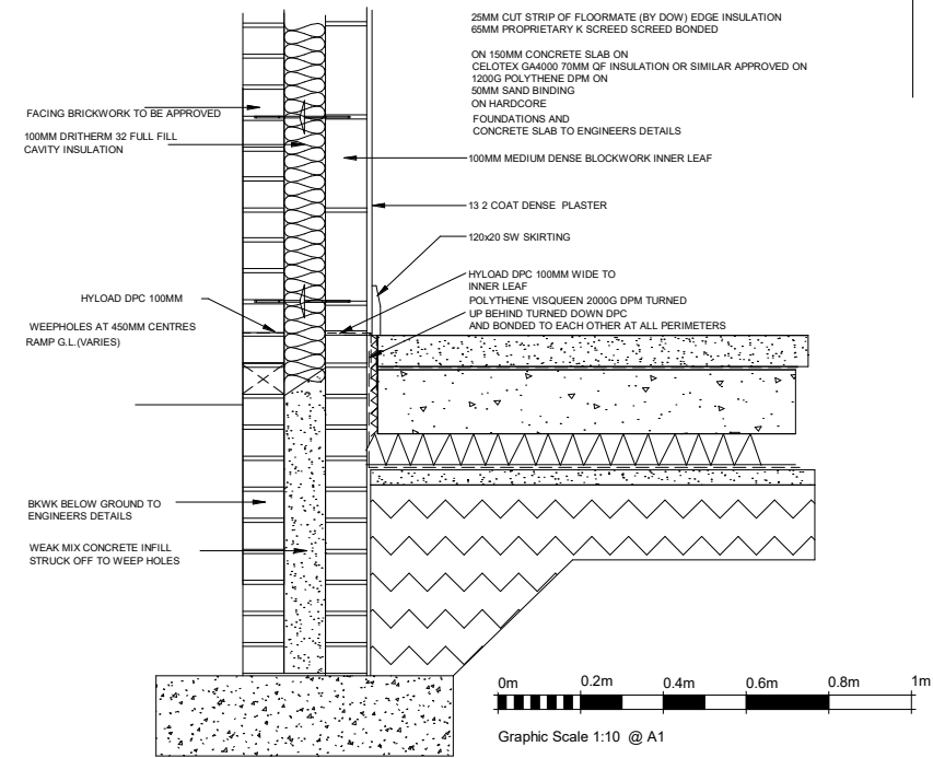
7 Slab Edge Detail
