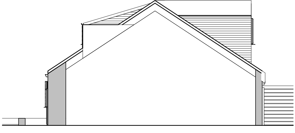
6 Existing Adjoined Elevation 1 : 100
