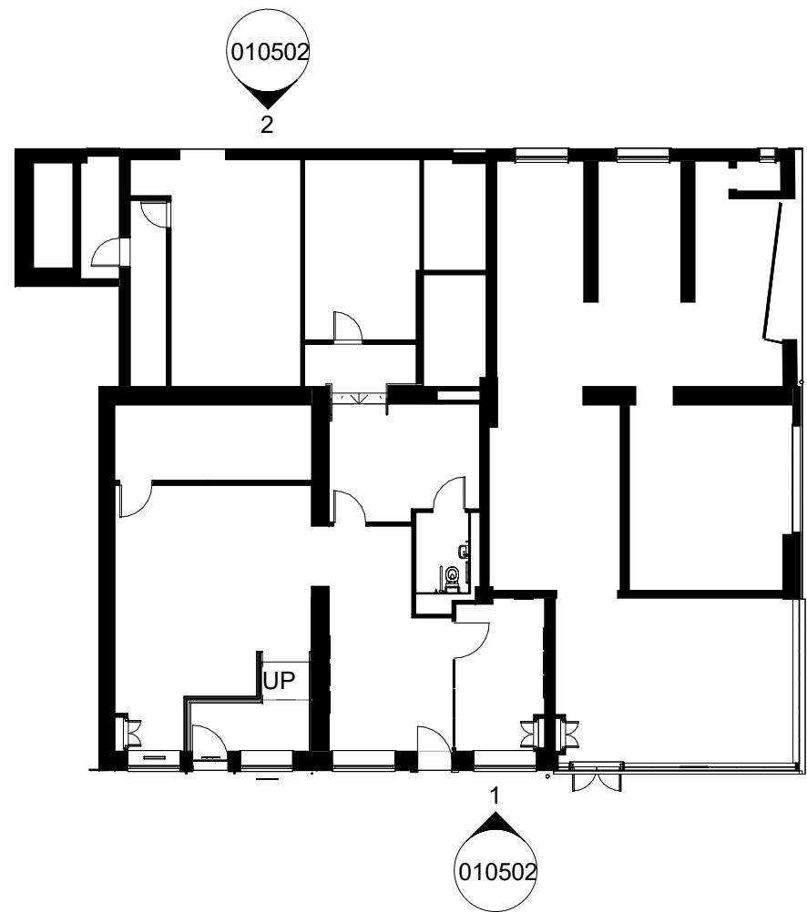
Key Plan 1 : 200
