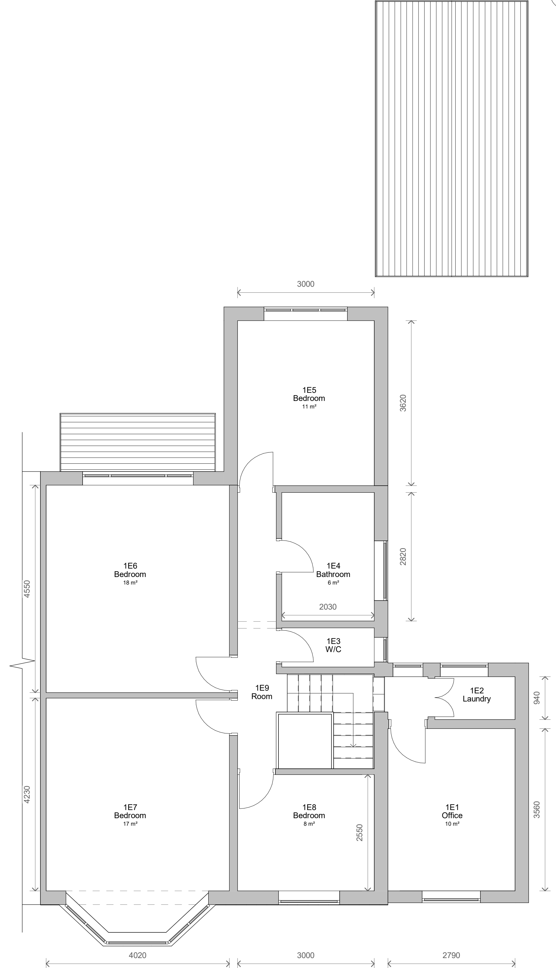
2 Level 1 - Existing 1 : 50
