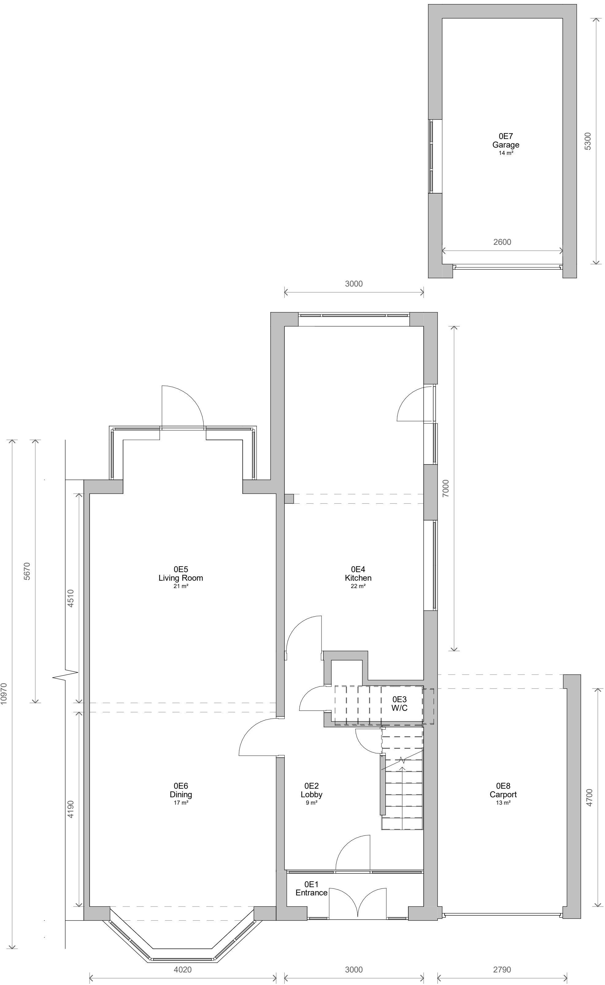
1 Level 0 - Existing 1 : 50
