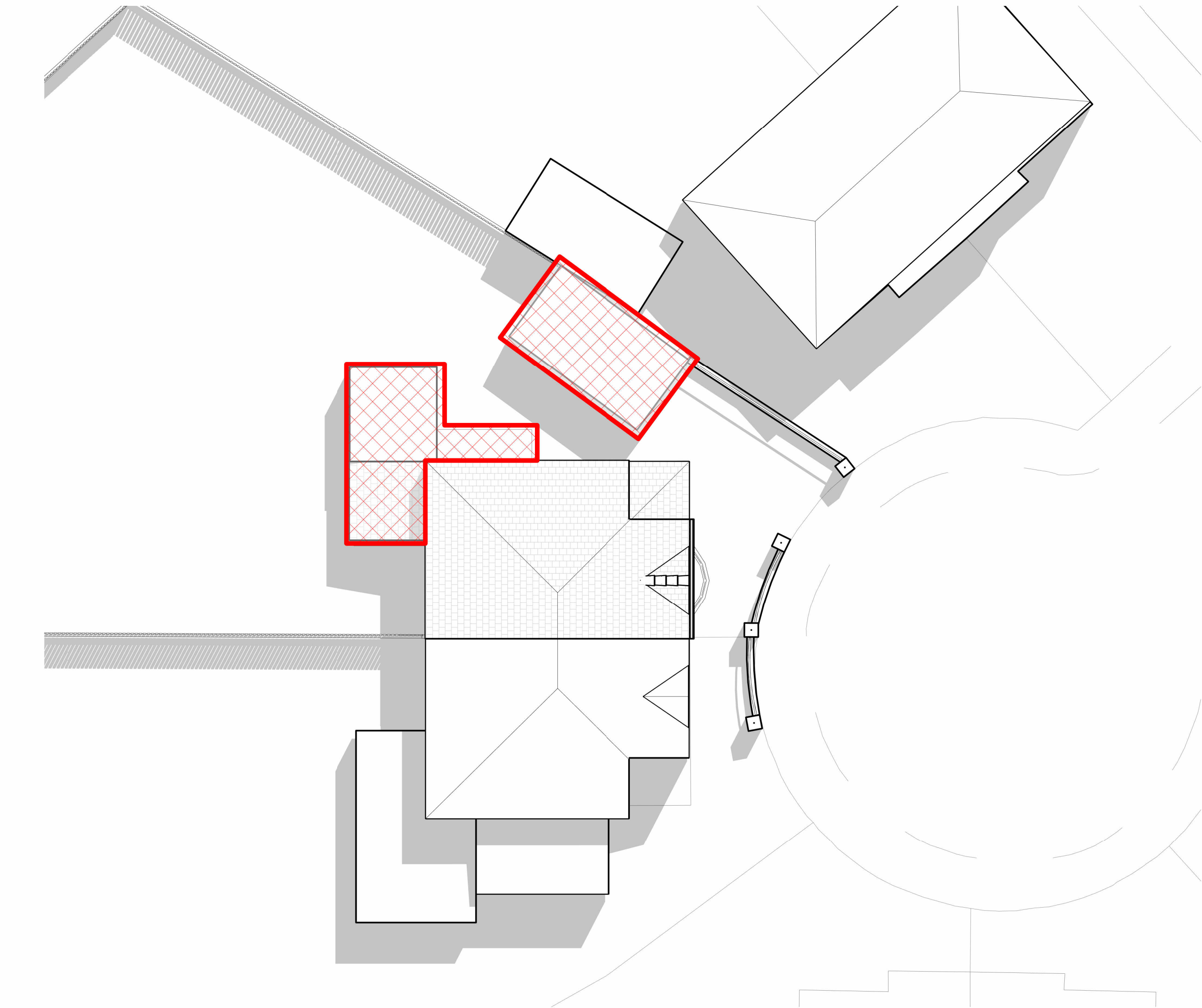
1 Demolition Plan 1 : 100
