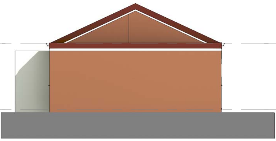
④ Left Side - Existing 1 : 100
