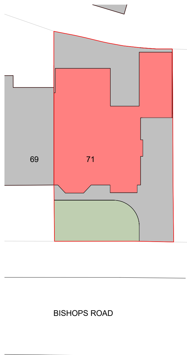
1 Site - Existing 1 : 200
