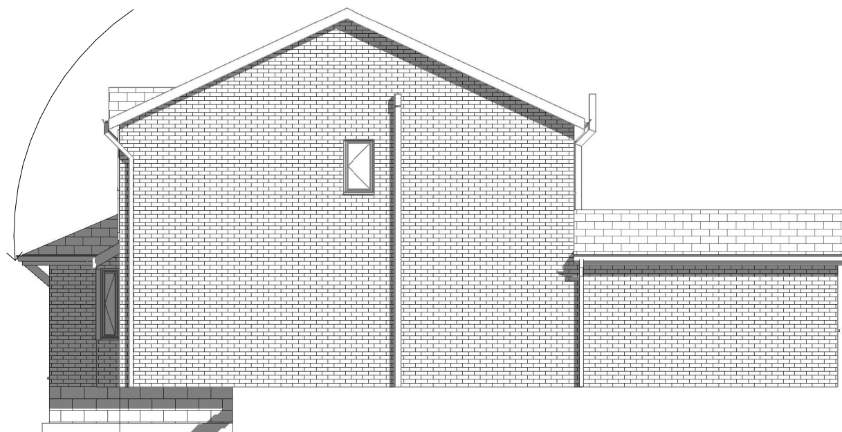
3 side 1 : 100
