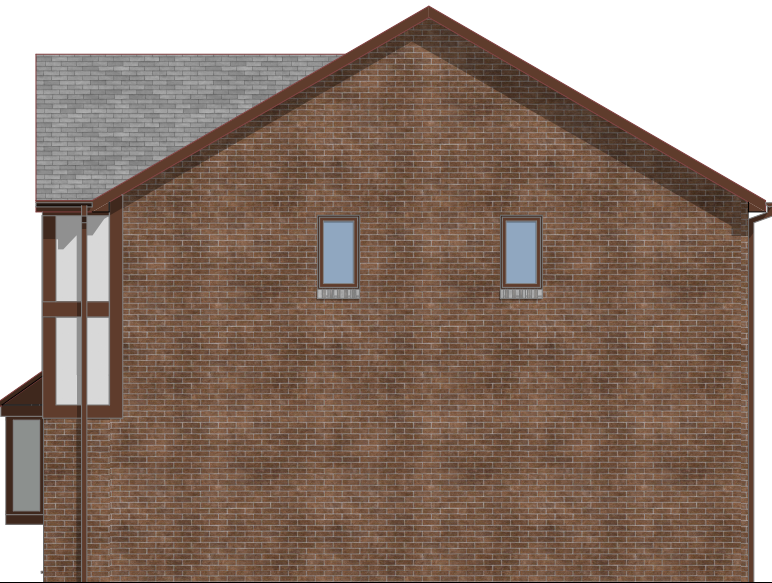
Side_2 elevation
