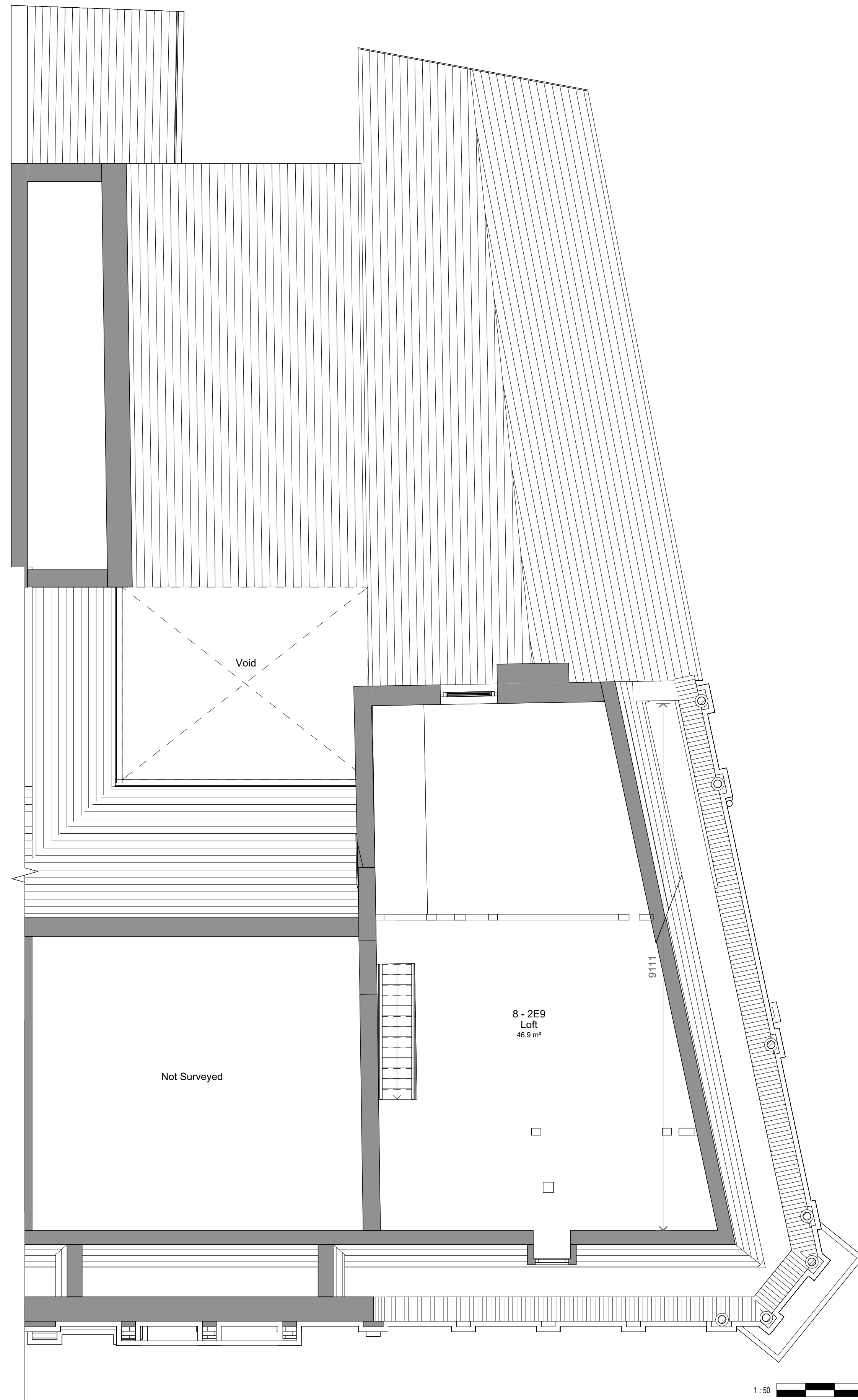
2 LEVEL 3 - Existing 1 : 50
