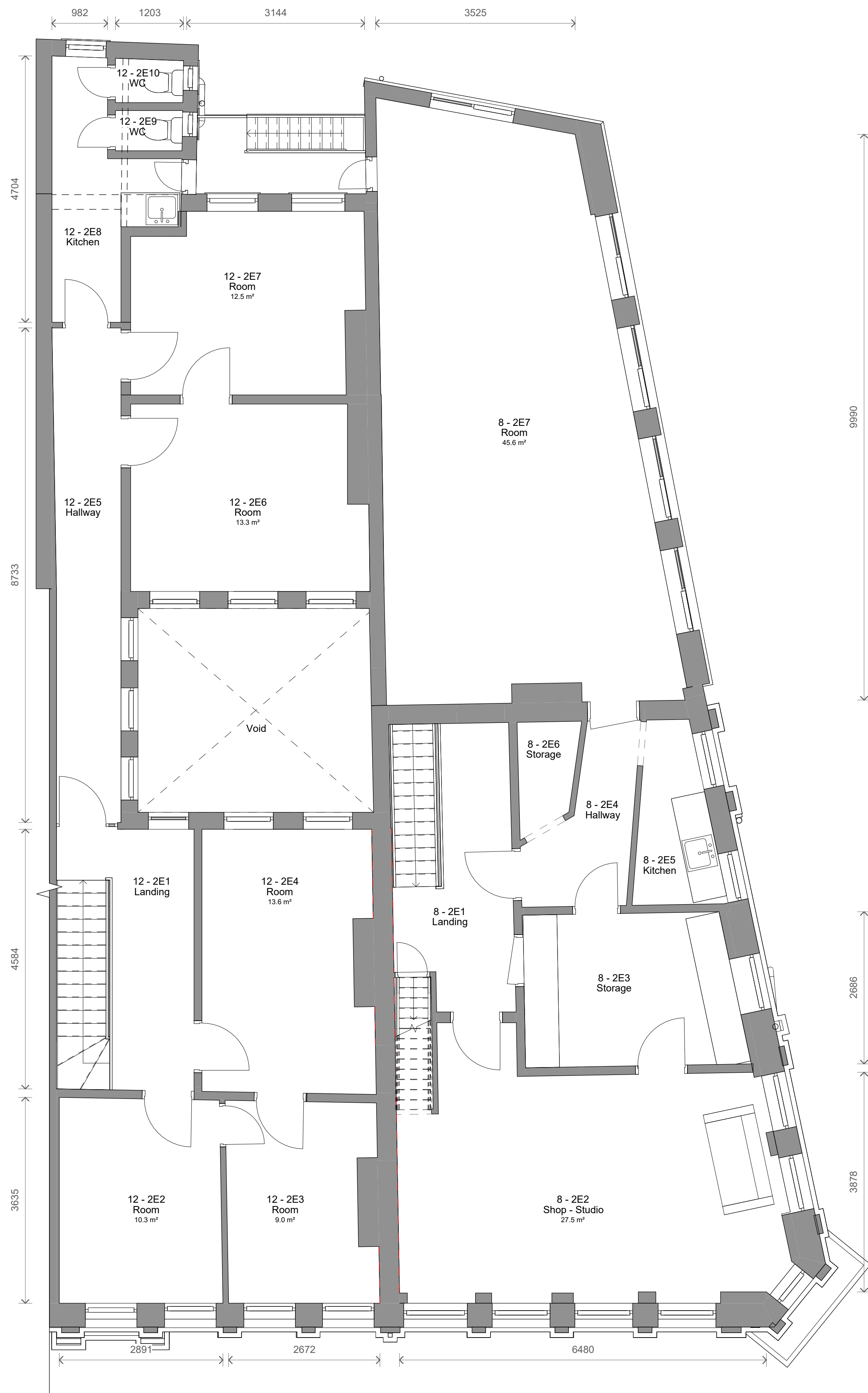
1 Level 2 - Existing 1 : 50
