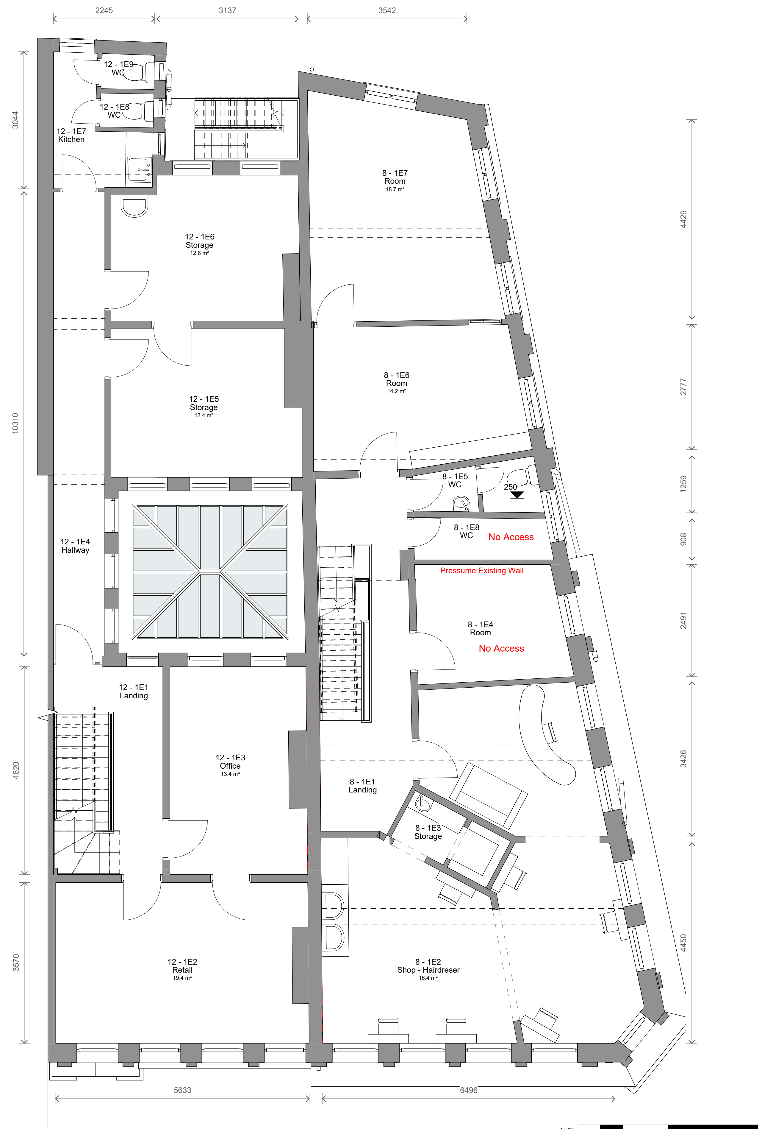
2 Level 1 - Existing 1 : 50
