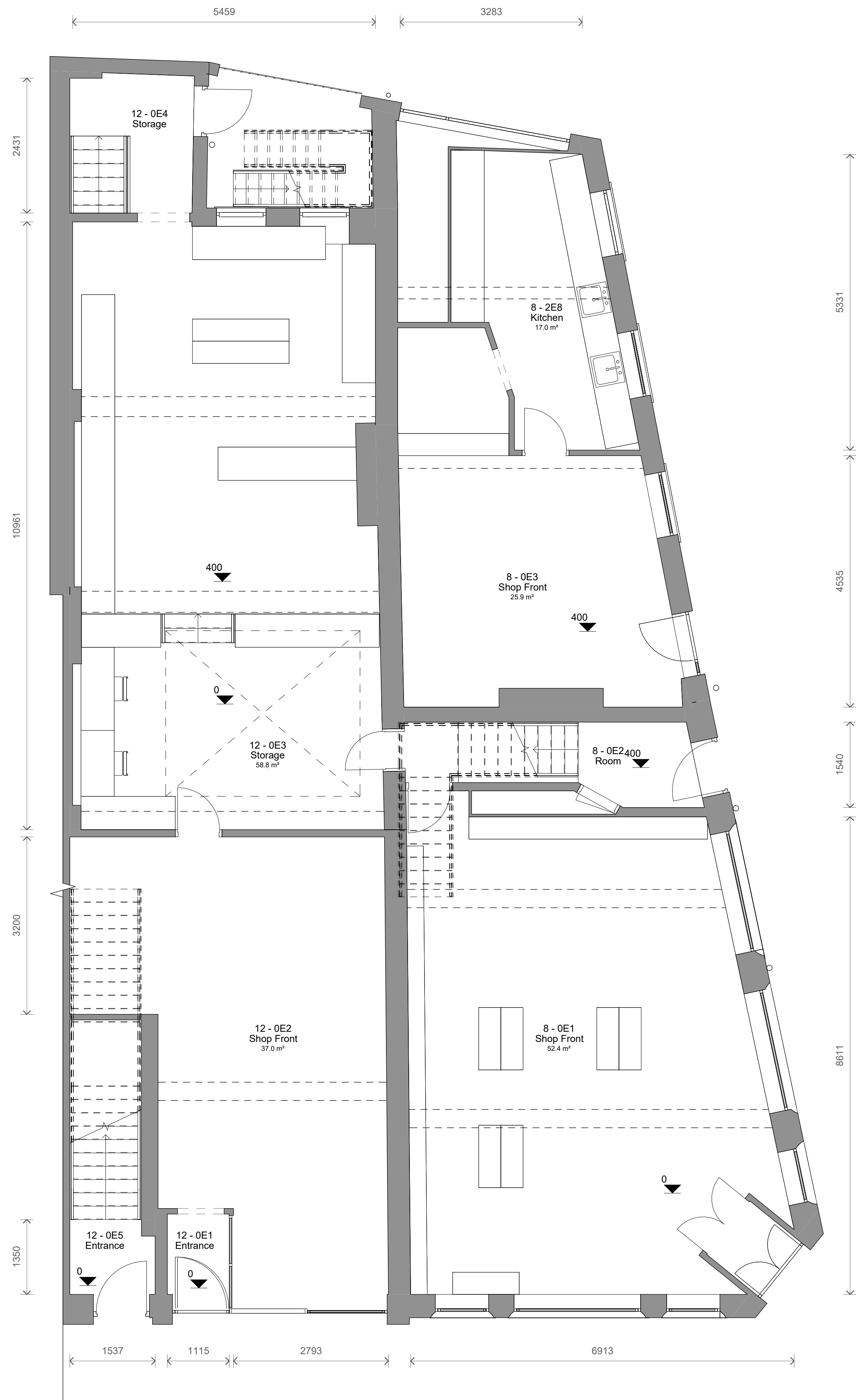
1 Level 0 - Existing 1 : 50
