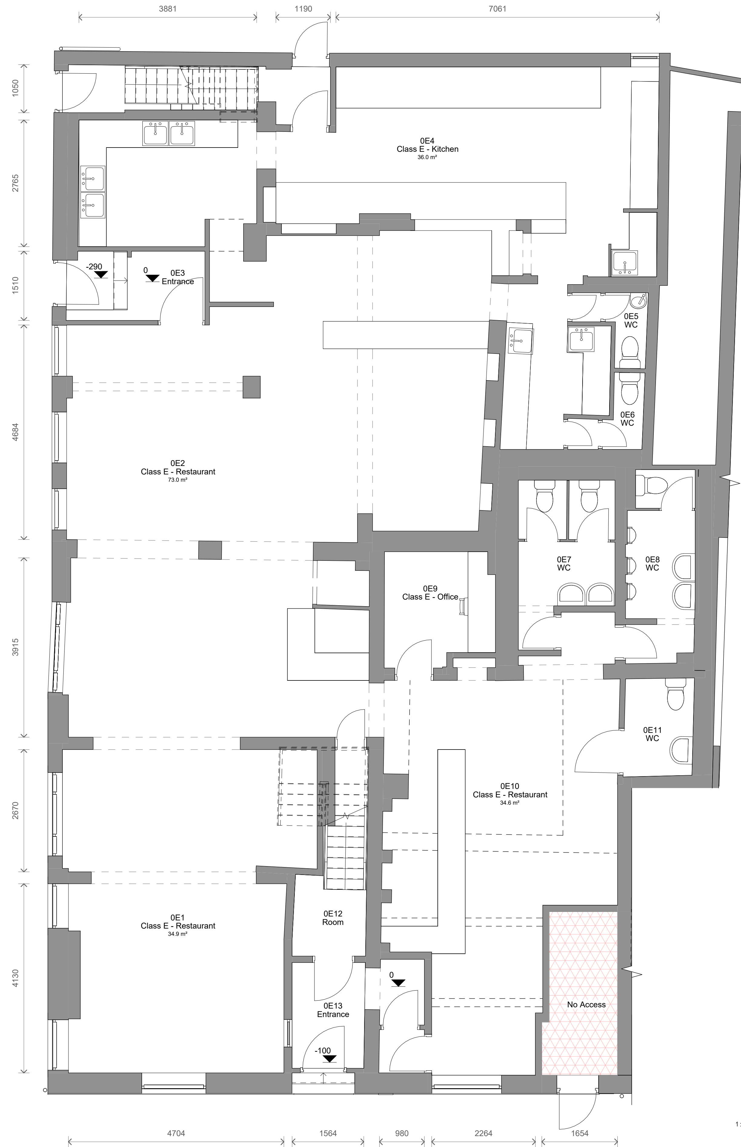
1 Level 0 - Existing 1 : 50
