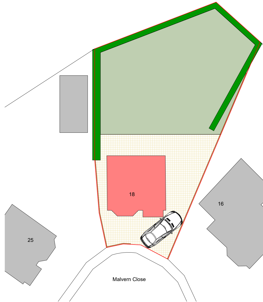
1 Site - Existing 1 : 200
