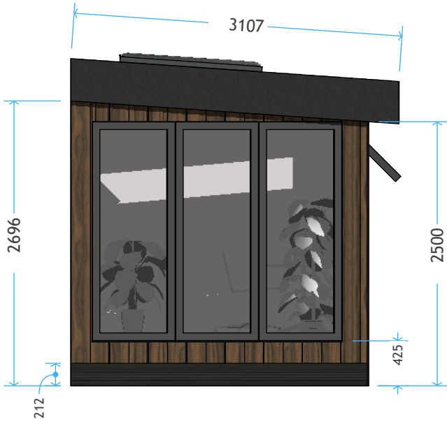
0 LH Elevation A03
