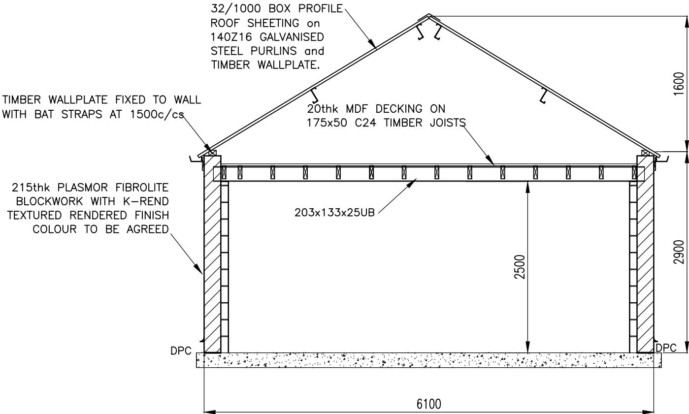
SECTION A-A 1:50
