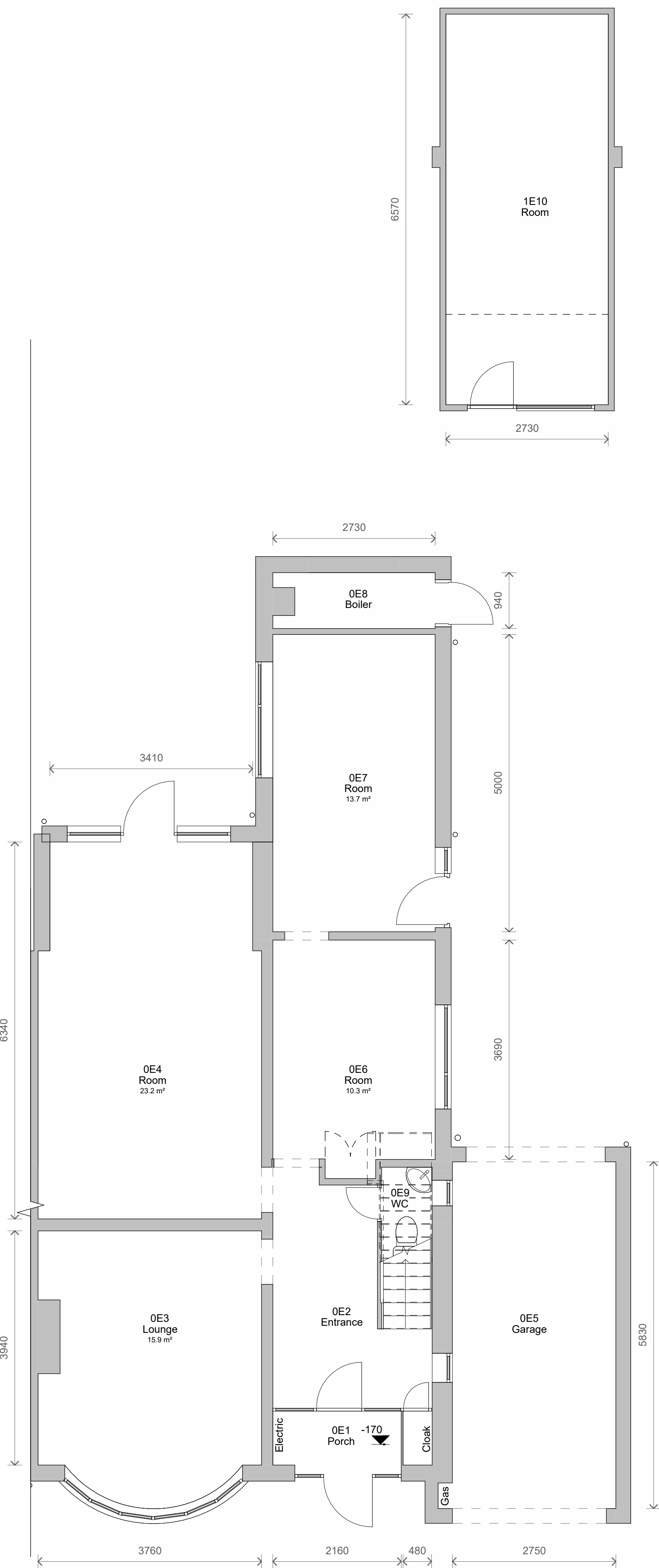
1 Level 0 - Existing 1 : 50
