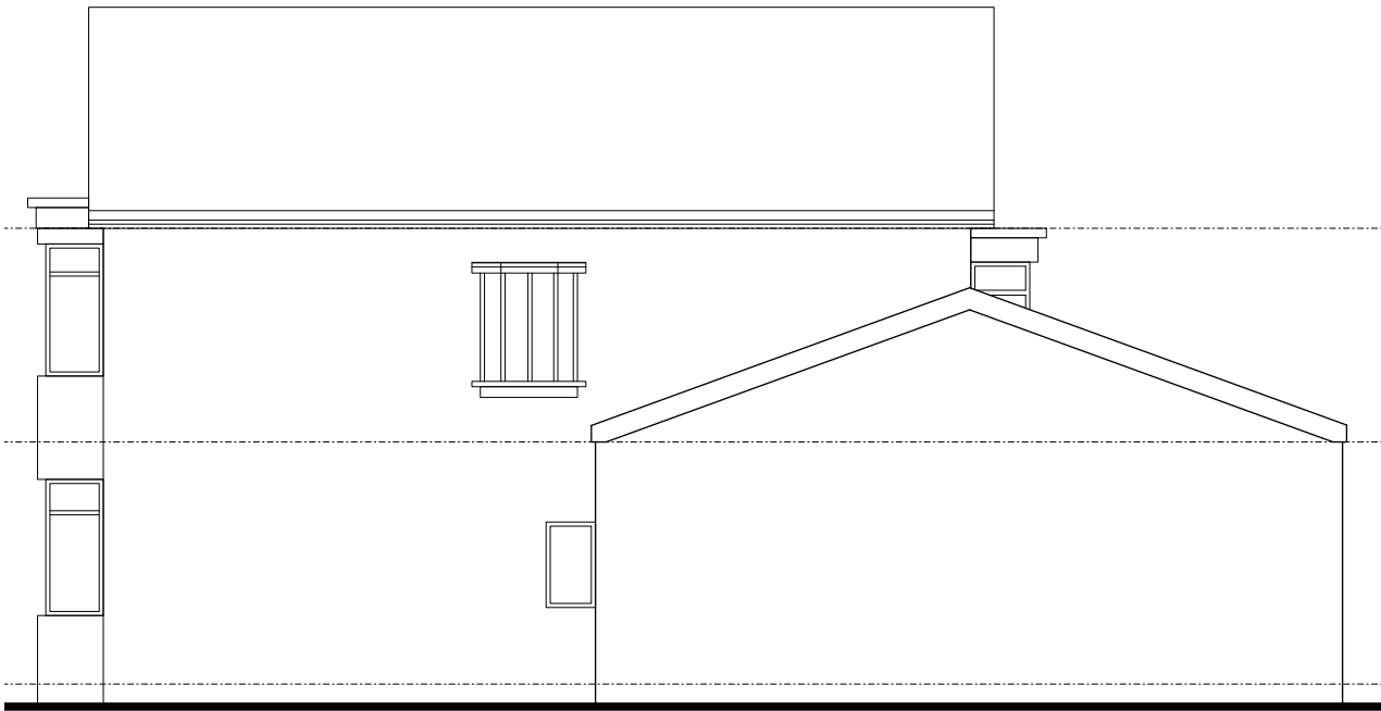
4 Existing Side Elevation 2 Scale: 1:100
