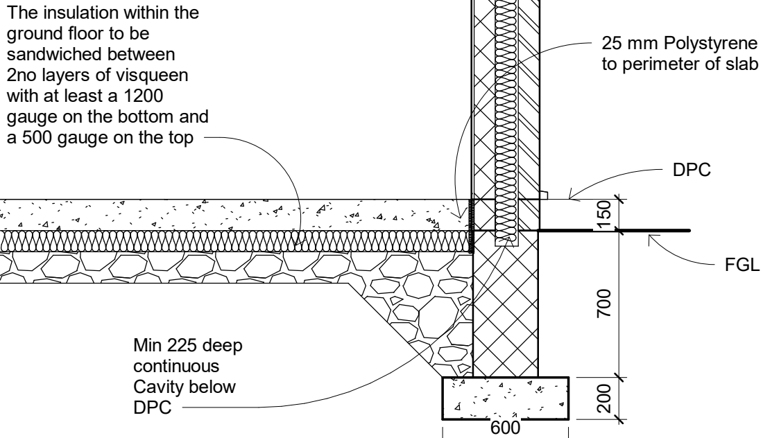
1 Section 1 - Callout 1 1 : 25
