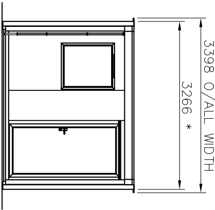
END ELEVATION
