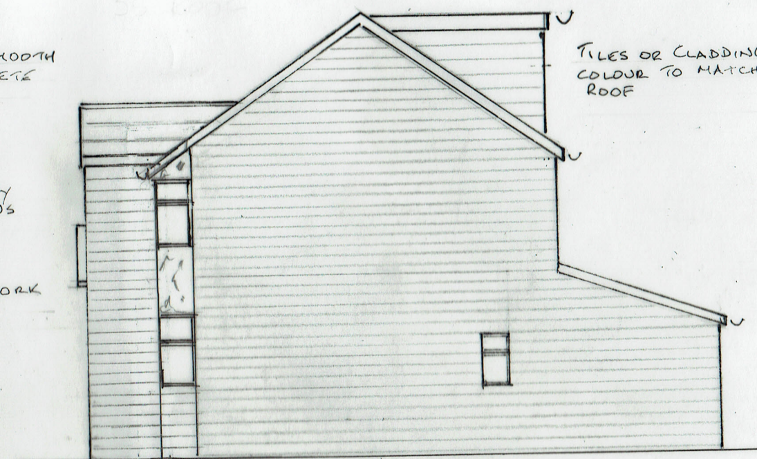
SIDE (NO. 3)
