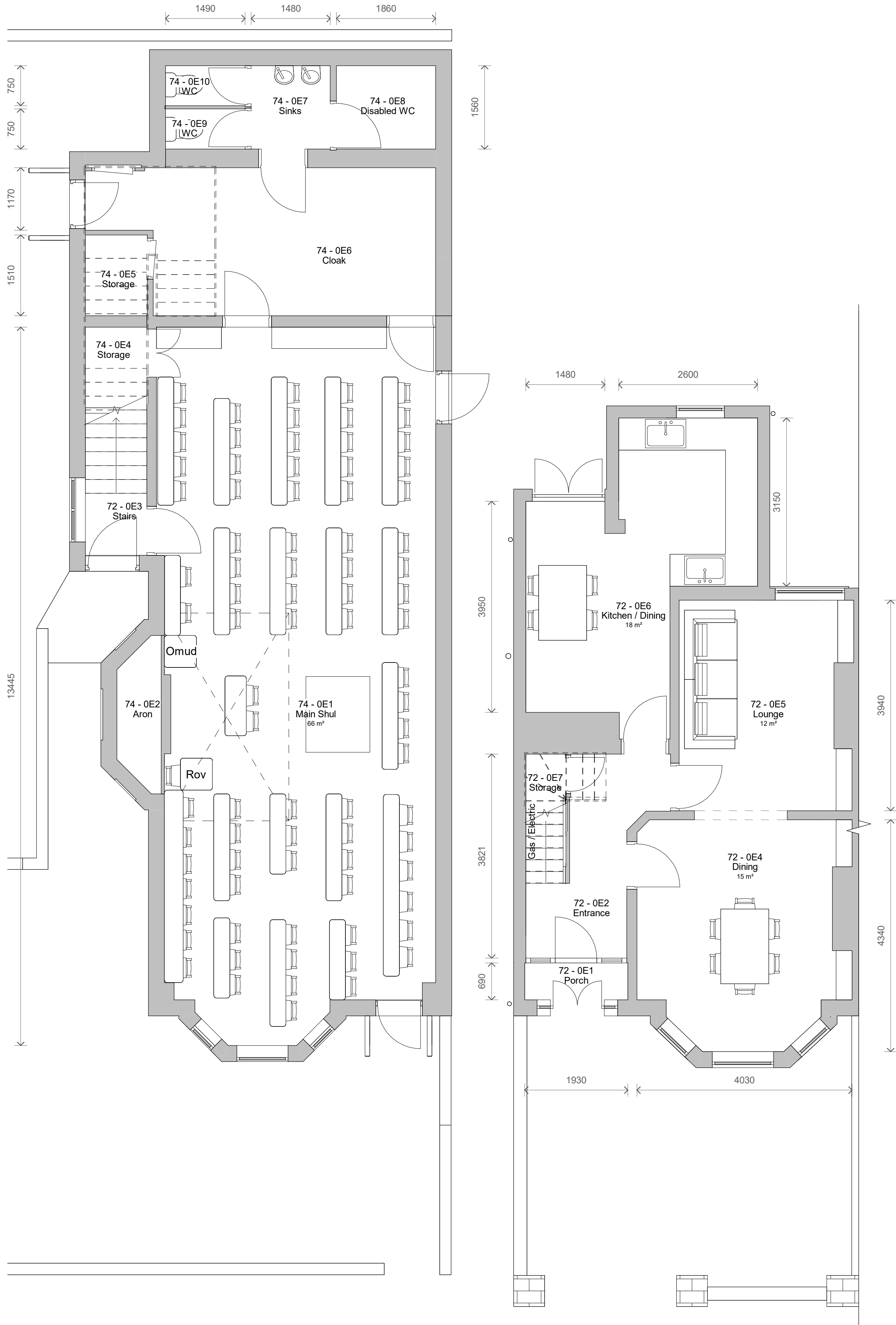
1 Level 0 - 72-74 - Existing 1 : 50
