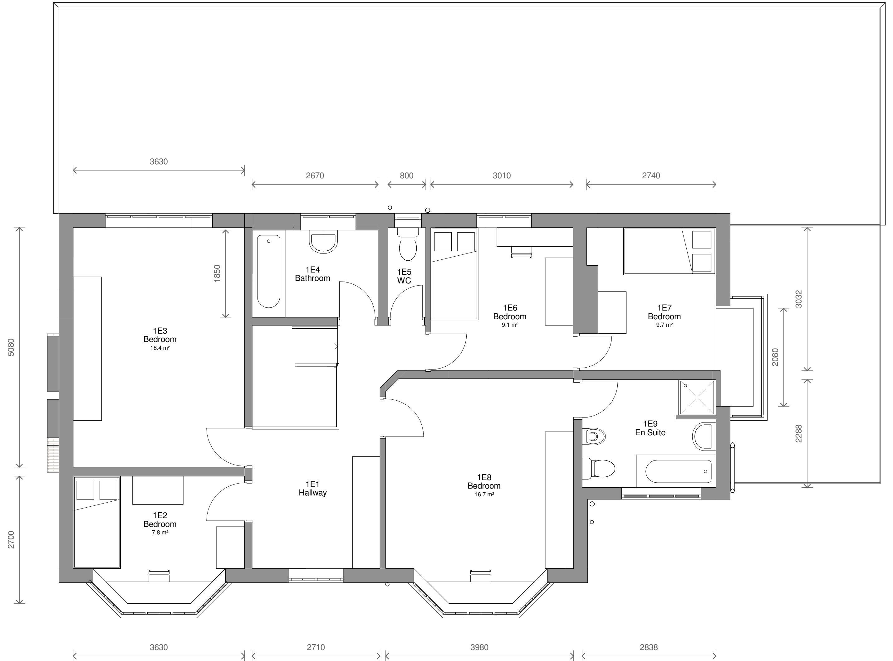
2 Level 1 - Existing 1 : 50
