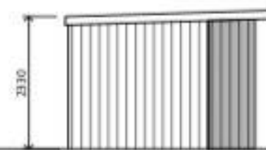
Side Elevation Scale 1:50 @ A1 1:100 @ A3
