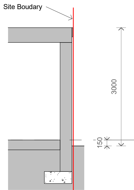
3 Section 1 1 : 50
