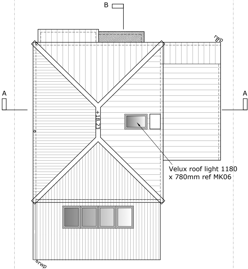
R O O F P L A N
