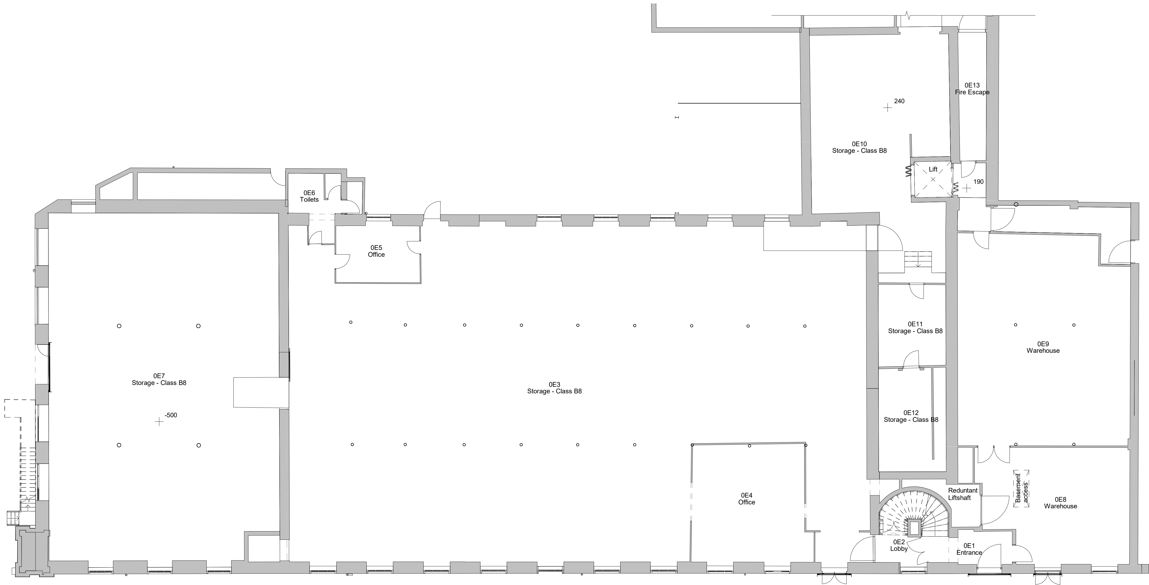
1 Level 0 - Existing 1 : 100
