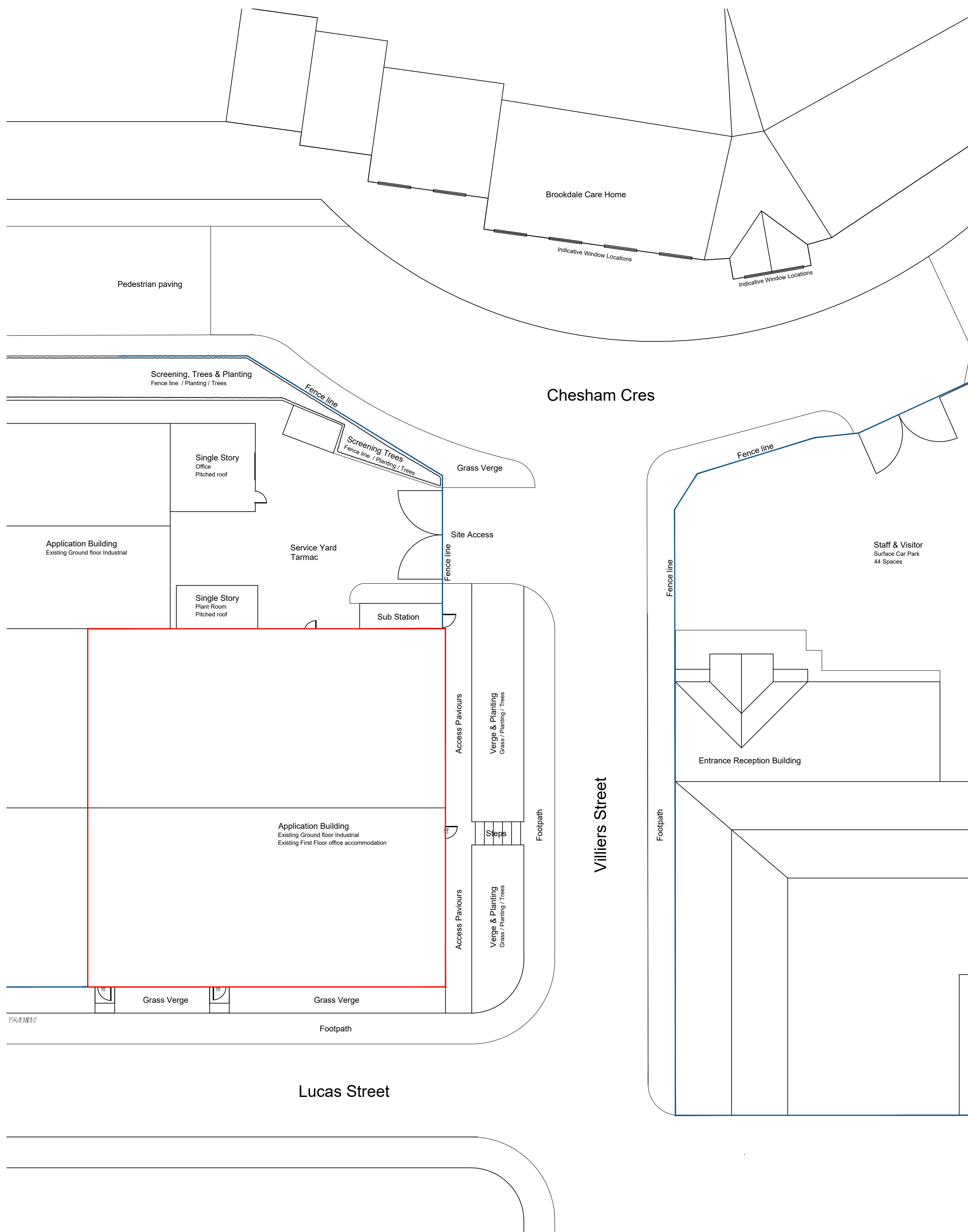
1 Existing Site Layout plan 1 : 200
