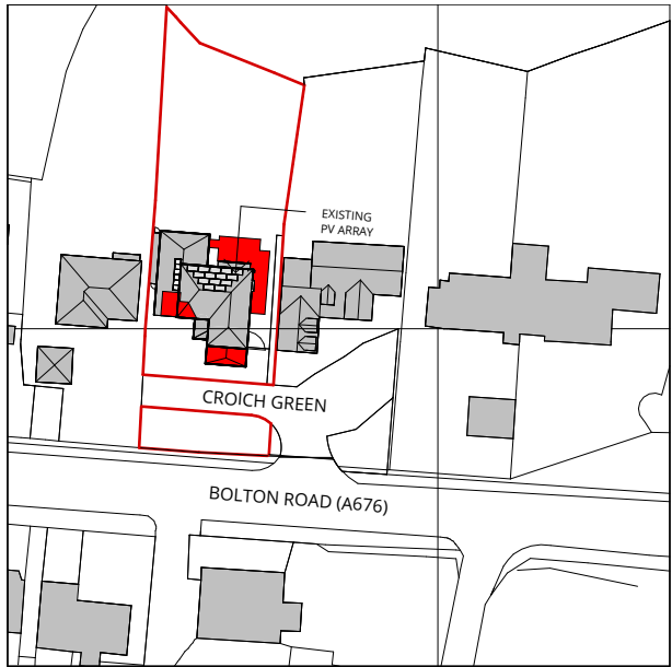
2 Block Plan 1 : 1250
