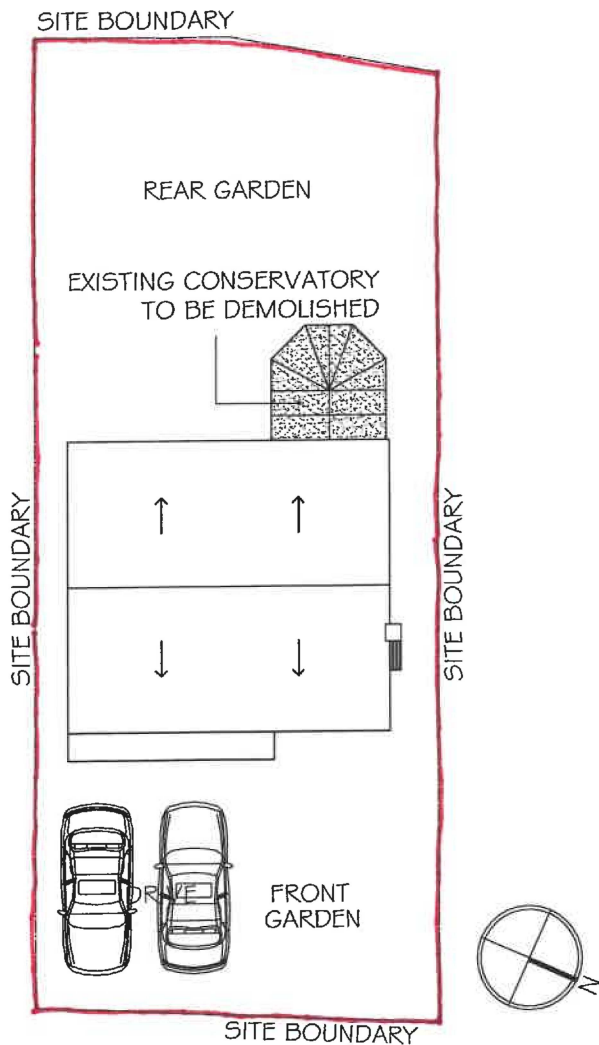
EXISTING SITE LAYOUT 1:200 @ A4
