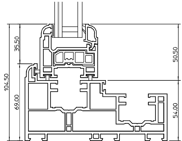
Top Jamb
