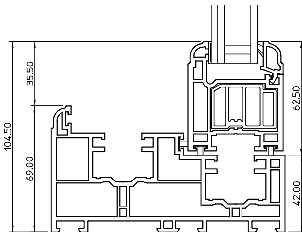
Side Jamb
