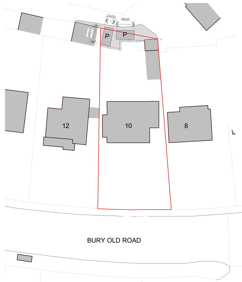
1 Site - Block Plan 1 : 500
