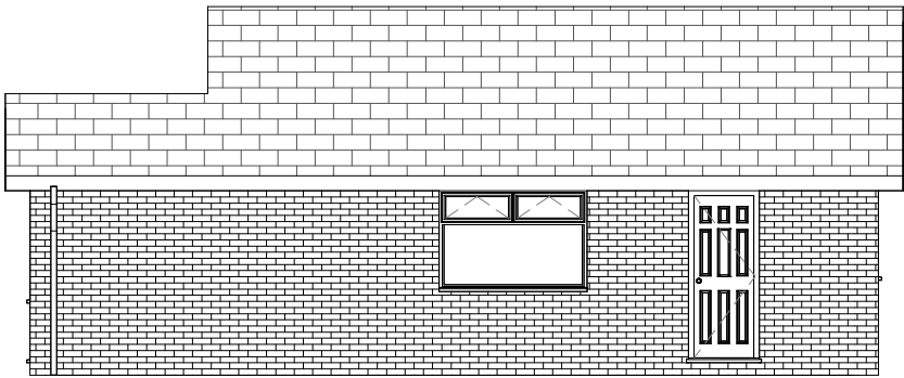
4 Garage Elevation 1 : 100
