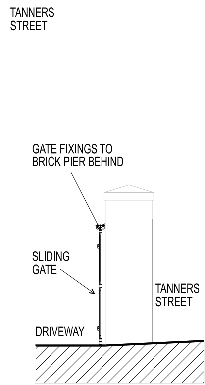
SECTION A-A
