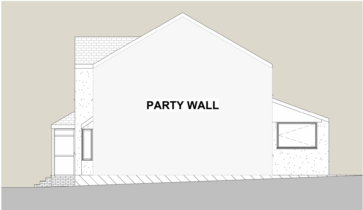
Ex RHS Elevation 1 : 100
