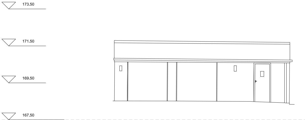
ELEVATION 1
