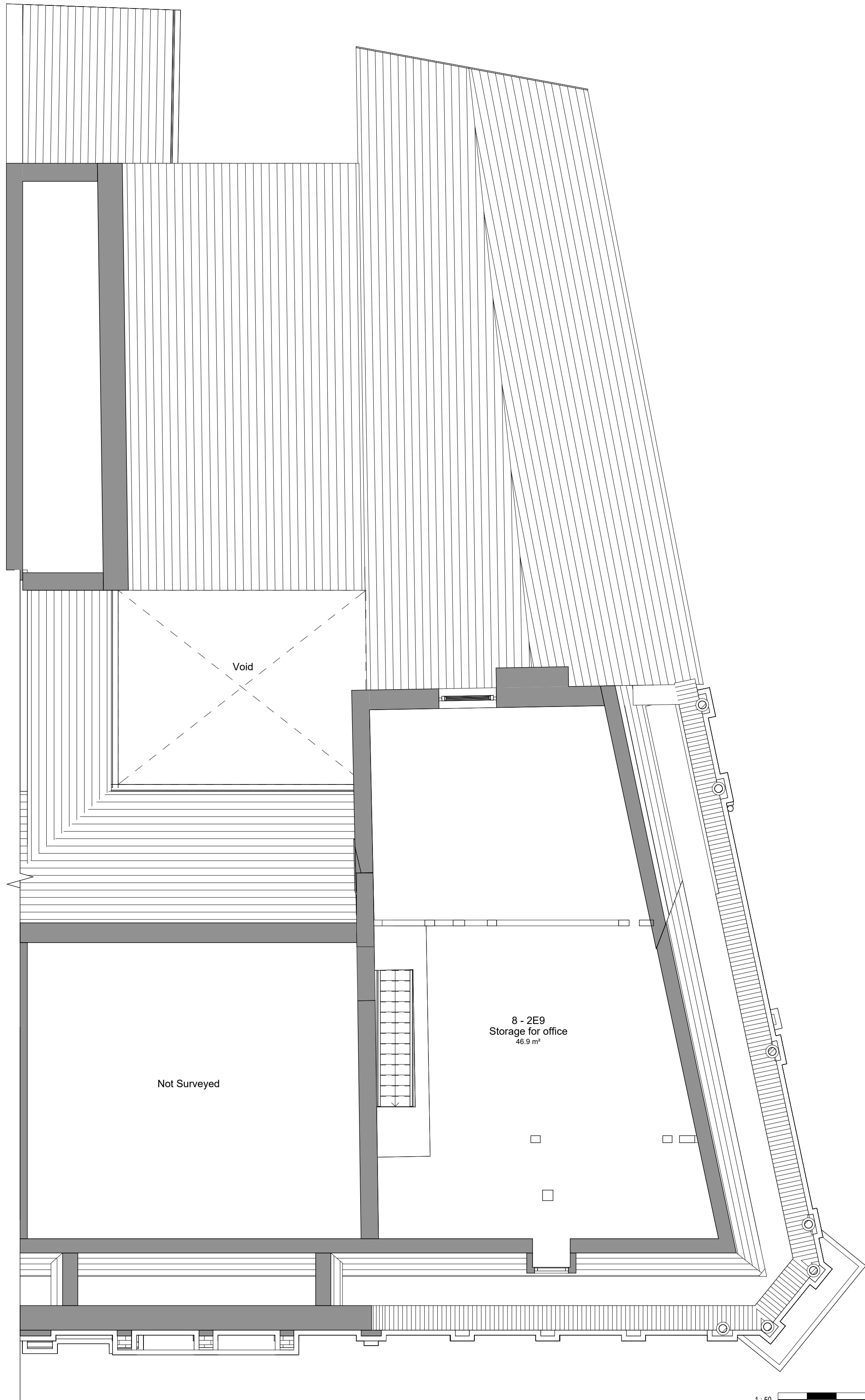
2 LEVEL 3 - Existing 1 : 50
