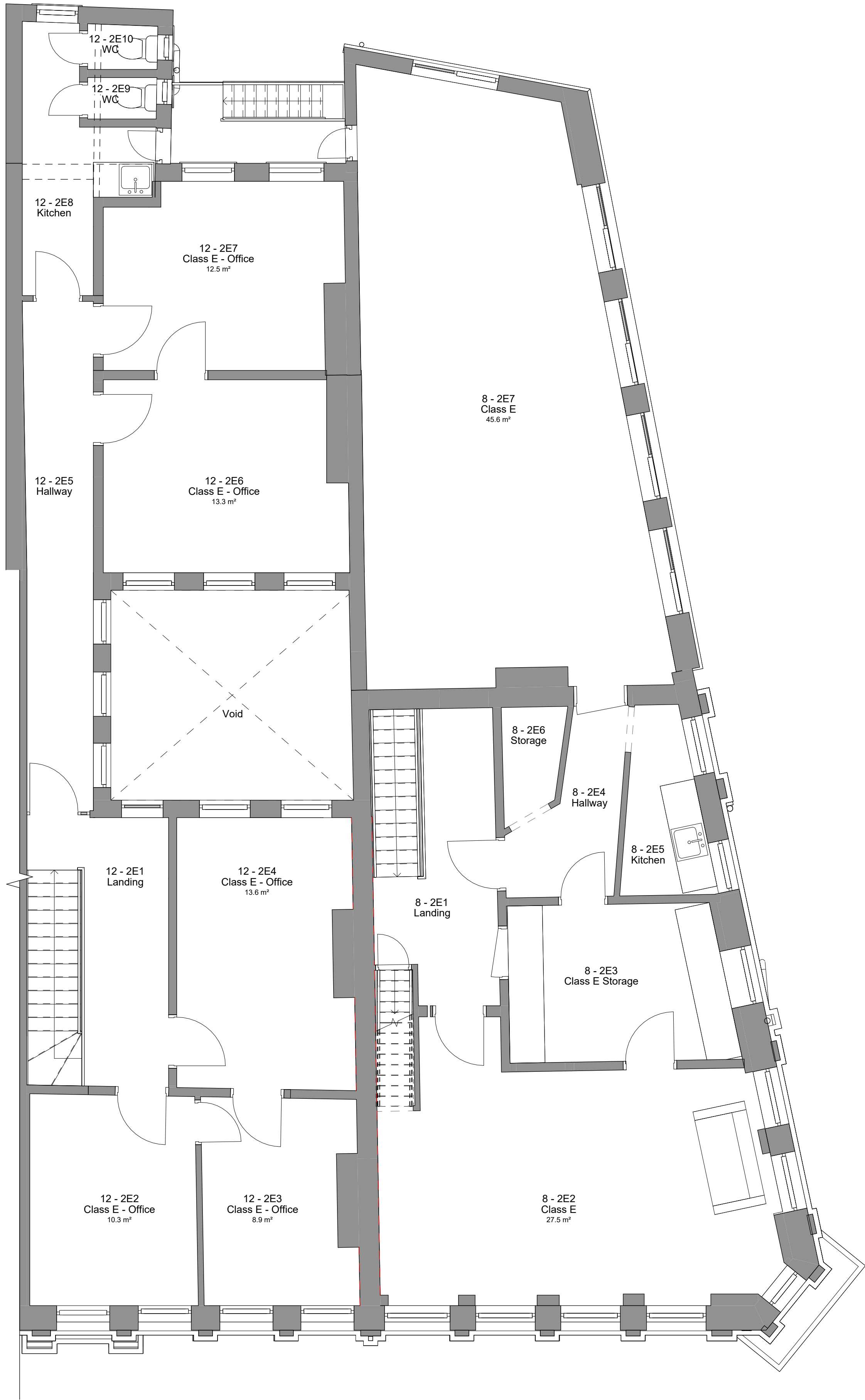
1 Level 2 - Existing 1 : 50
