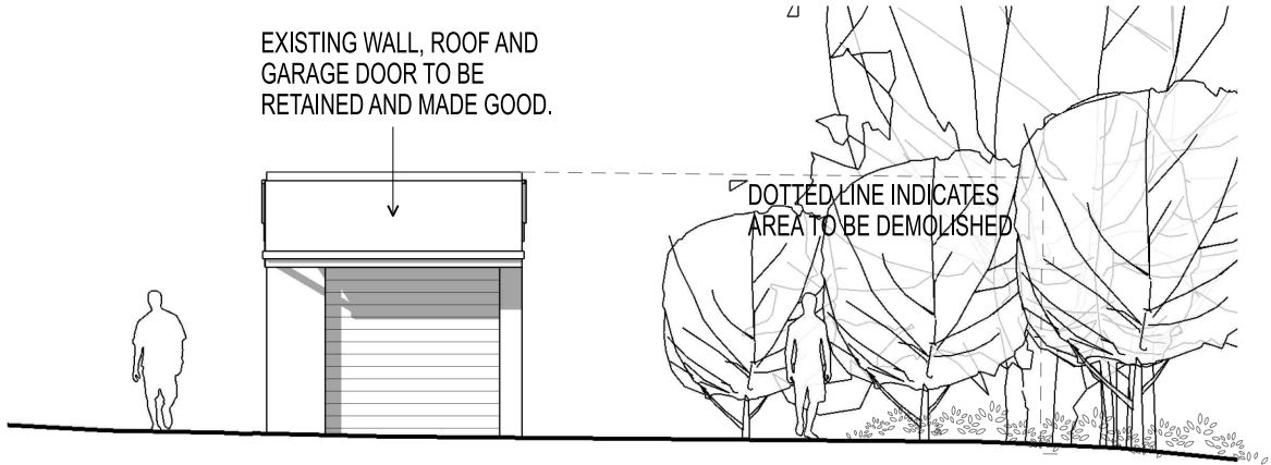
datum +67.50 ELEVATION 1
