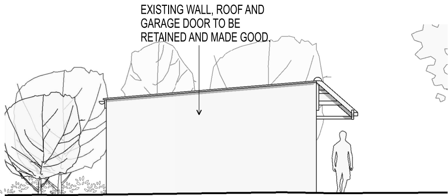
datum +67.50 ELEVATION 2
