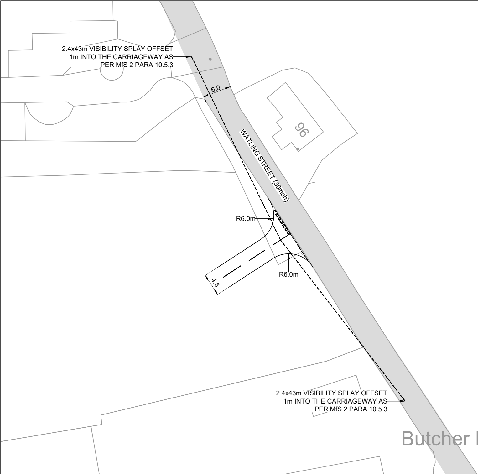
SITE LAYOUT NTS
