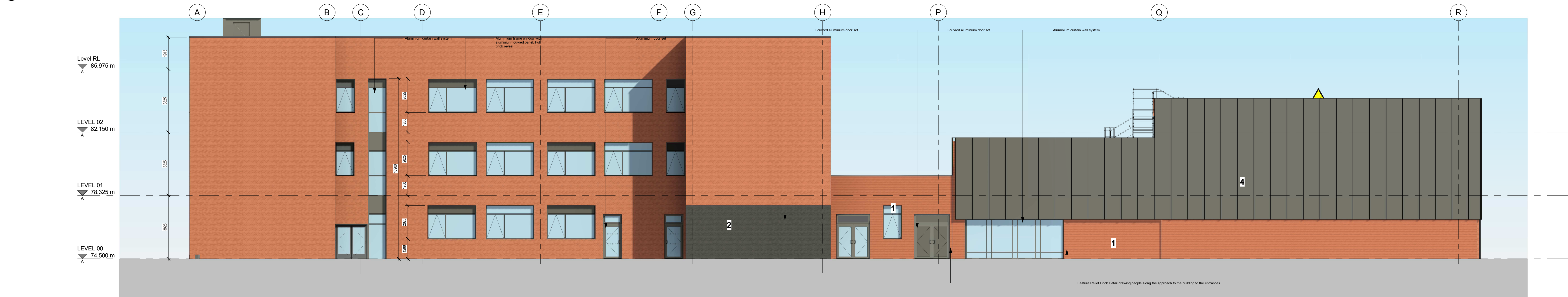
4 ALL WEST 1 : 100
