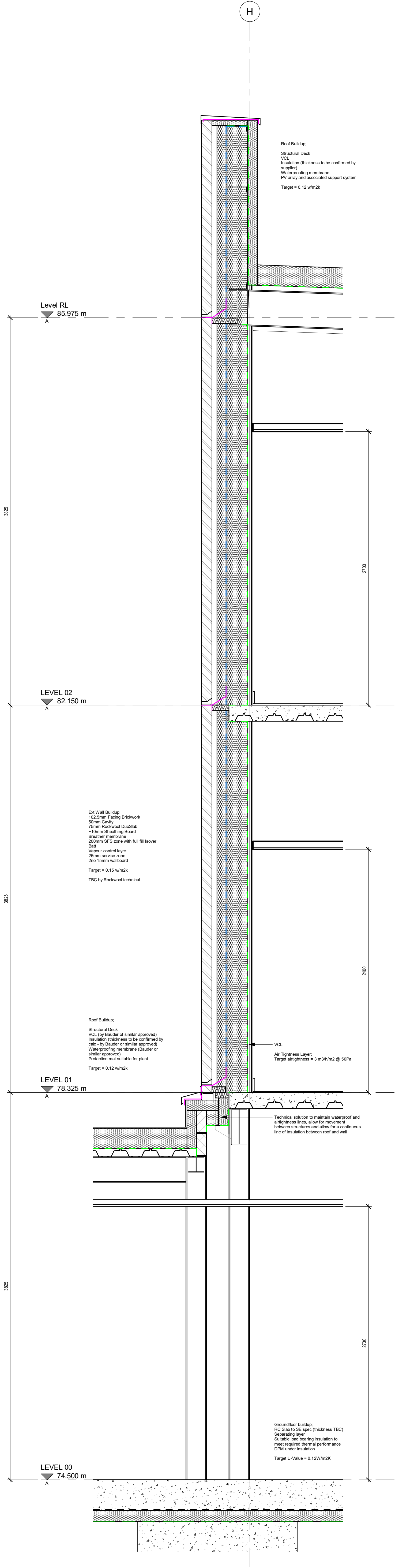
1.2 Section 1.2 1 : 20
